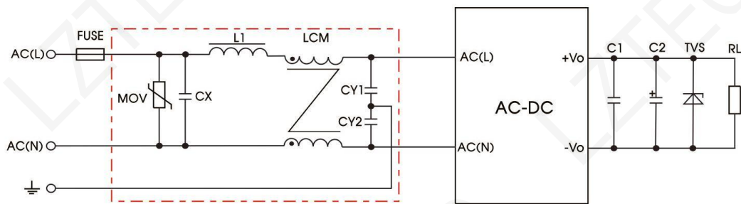
EMC 推荐电路
