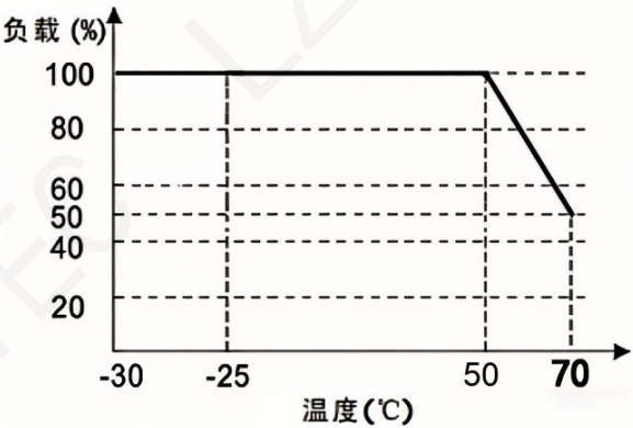
温度与负载关系图 TEMPERATURE VS. LOAD
