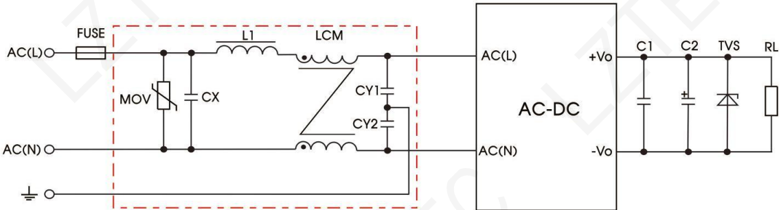
EMC 推荐电路
